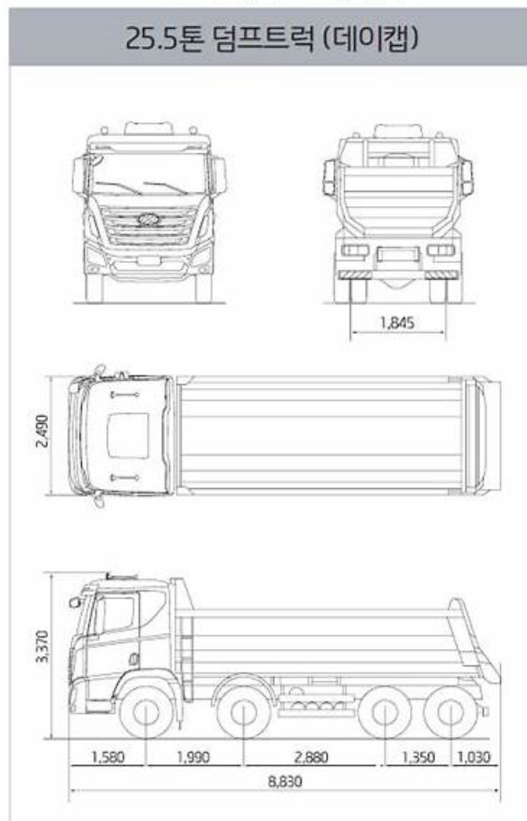
25.5톤 덤프 (데이캡)
